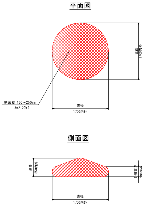
袋詰め玉石構造図 S=1:30 (参考図)
